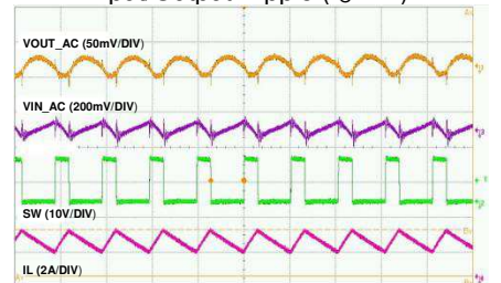
Input/Output Ripple (I O =2A)
