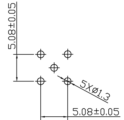
安装插板开孔尺寸
