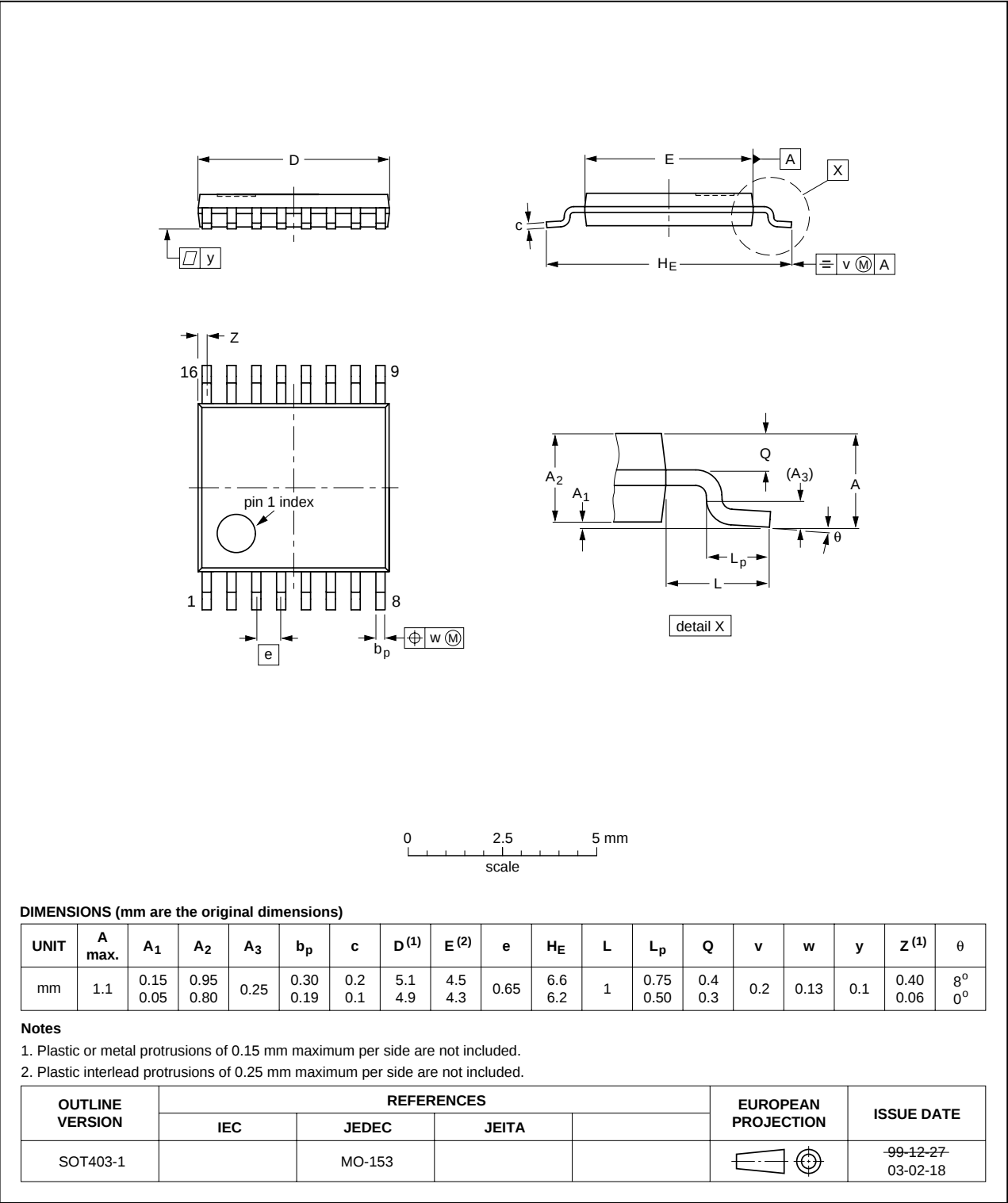
Fig 29. SOT403-1 (TSSOP16).
