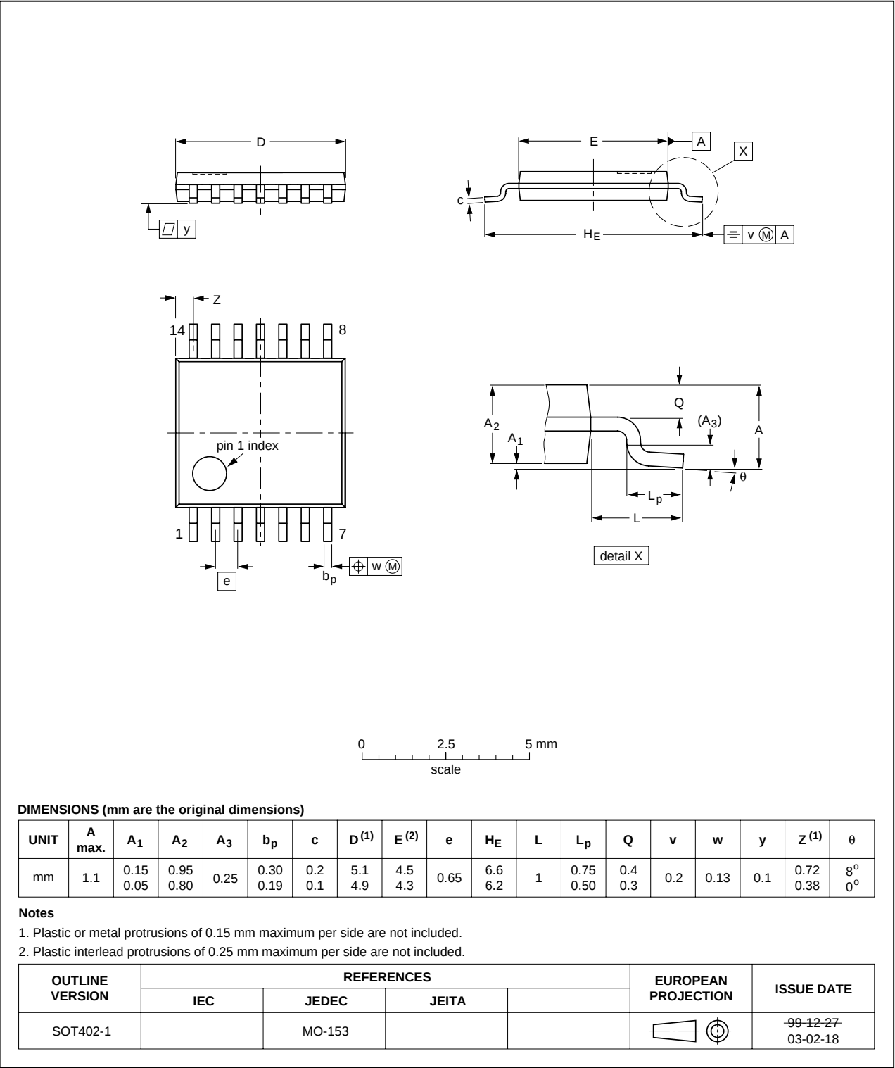
Fig 28. SOT402-1 (TSSOP14).
